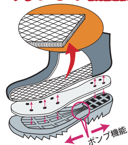
▲ エアサイクル構造
